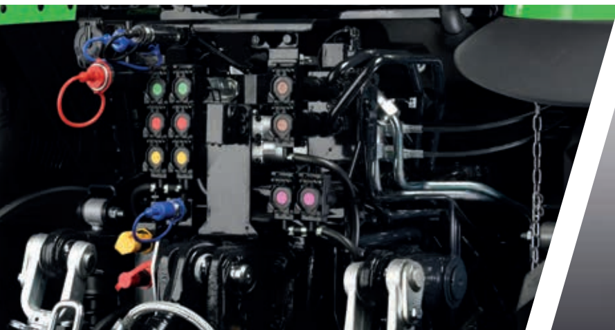
> Hasta 10 salidas traseras.
