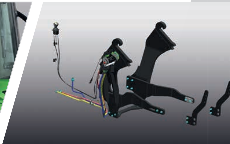
> El Ready Kit incluye, además, un circuito hidráulico específico para trabajar con un elevador y un joystick dedicado, montado junto al asiento del conductor.
