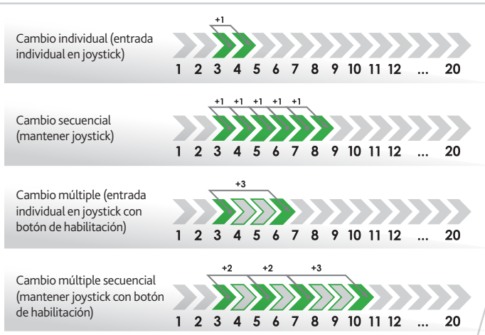
> Modos de cambio.
