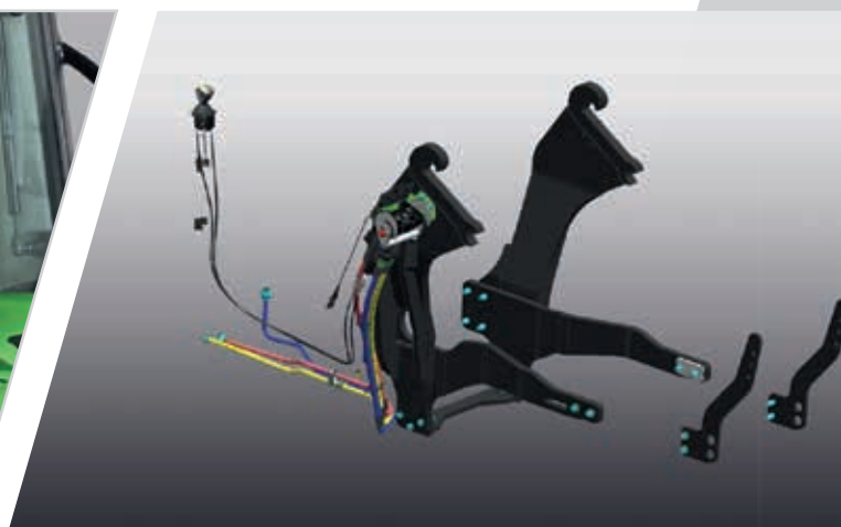
> Le Ready Kit comprend également un circuit hydraulique spécifique pour travailler avec un relevage et un joystick de commande dédié à proximité du siège conducteur.
