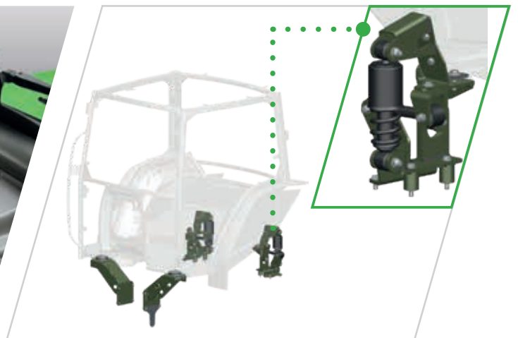
> Suspension mécanique cabine.
