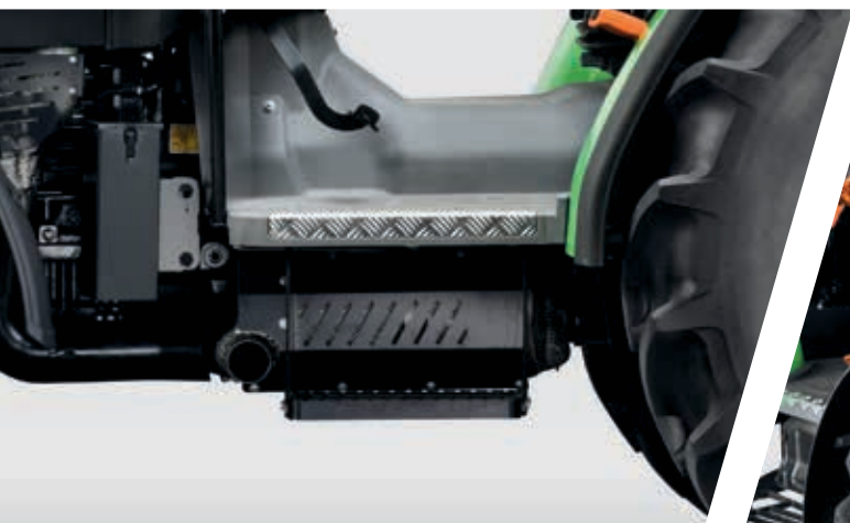
> Volledig geïntegreerd EAT-systeem. SCR en DPF die de hoogte van de spatborden en de afmetingen van de motorkap niet beïnvloeden.
