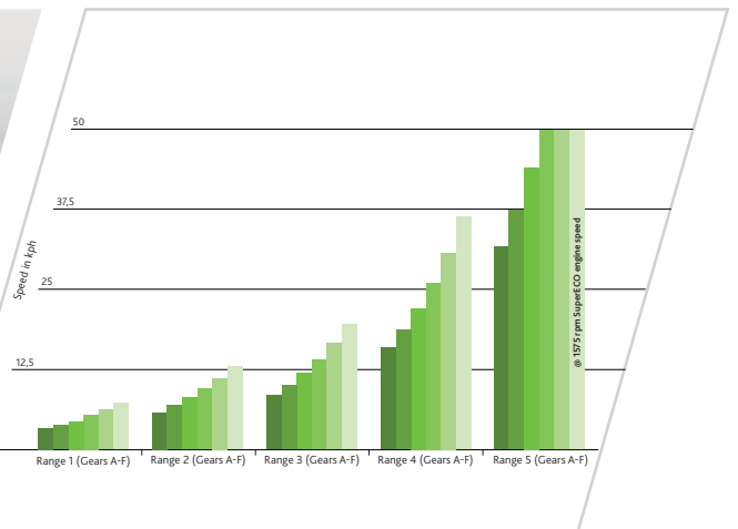
> Velocidades RCshift: sobreposição excepcional das diferentes gamas e superECO de 50 km/h para máxima eficiência de combustível (rpm do motor com o tamanho máximo dos pneus).
