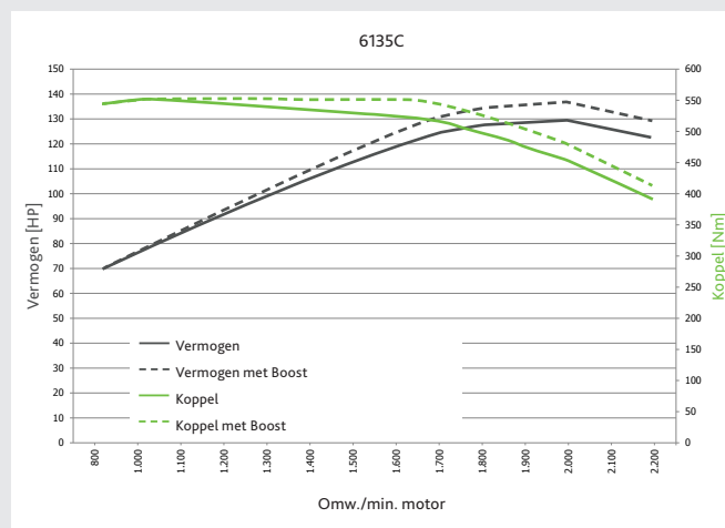
6135 C FARMotion motorgegevens.
