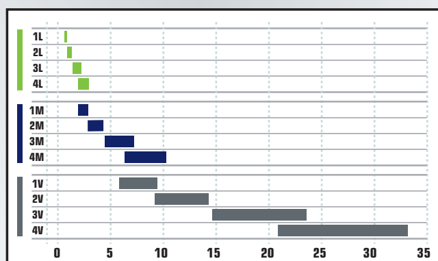
Für alle Arbeiten passend abgestuft: Das Synchrosplit-Getriebe.
